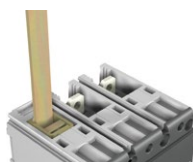
Prise FB avec jeux de barres souples
