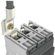
Prise ES se terminant par une cosse
