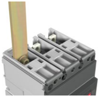
Prise F avec jeu de barres
