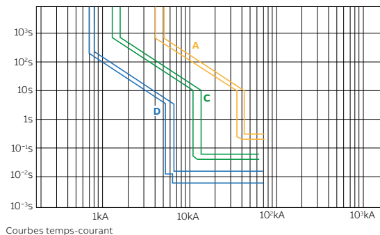
Fig. 2 – Seuils de protection en fonctionnement sur réseau
