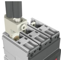
Prise externe FC-CuAl avec câble
