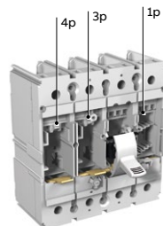
Disjoncteur tétrapolaire
