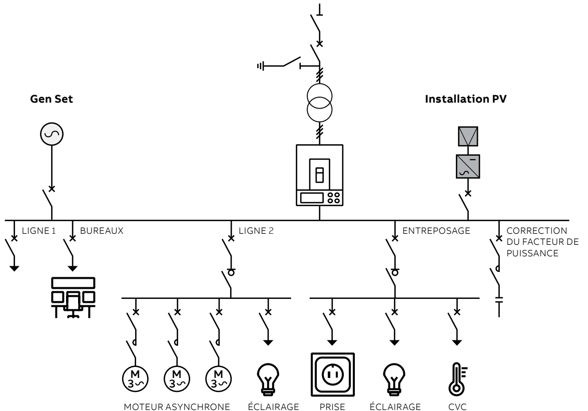
Application typique de délestage
