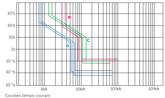
Fig. 3 – Seuils de protection en fonctionnement îloté
